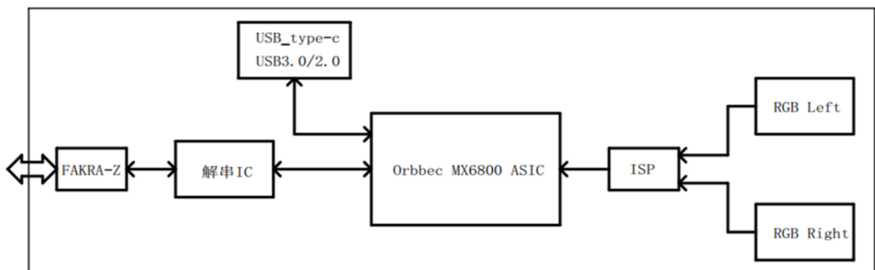
图 4-3-1 Gemini 305g 相机系统框图
