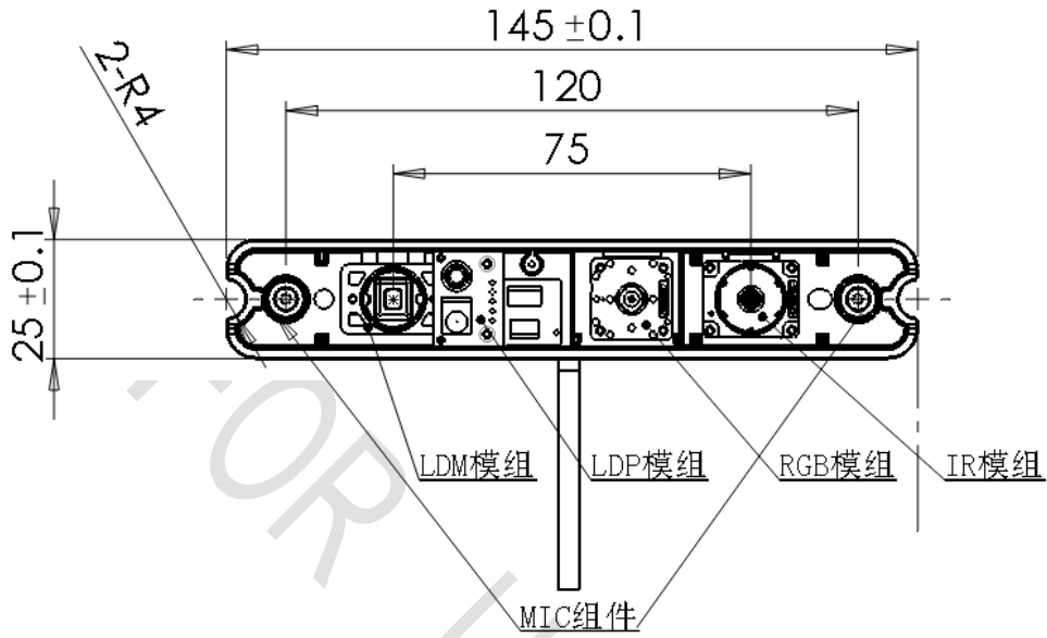
图 3 产品正视
