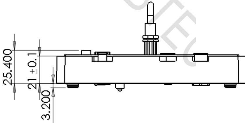
图 4 产品侧视
